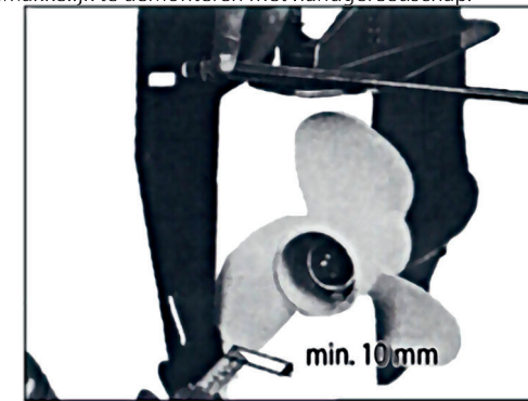
Fig. 4 De afstand tussen het roerblad en de schroef dient ca. 2,5 cm te bedragen. Dit is geen vereiste en kan per motor of staartstuk variëren. Minder dan 1 cm wordt afgeraden.
