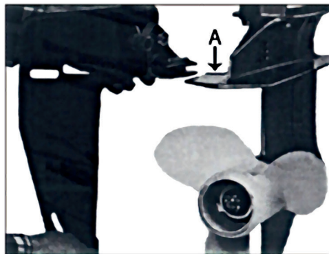
Fig. 2 Leg, indien nodig, vulplaatje A op de bovenzijde van de cavatieplaat.
