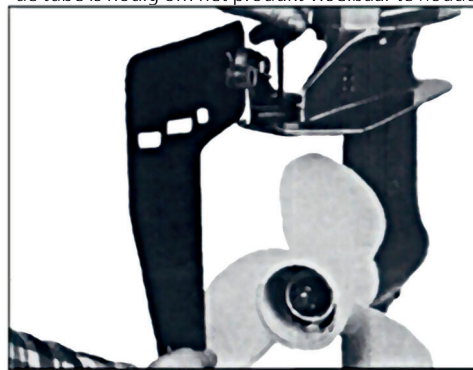
Fig. 3 Schuif het roerblad met de bracket over de cavatieplaat en het eventueel aanwezige vulplaatje, totdat deze stuikt. Bevestig het roerblad "los-vast" aan de cavatieplaat, door de bovenste en onderste stelschroeven, gelijmatig aan te draaien. Een slag onder, een slag boven, enz. Het roerblad dien parallel aan de hartlijn van de motor te worden gemonteerd.
